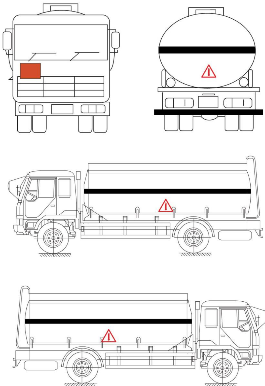
图 B.8 高温物质标记悬挂位置示意
